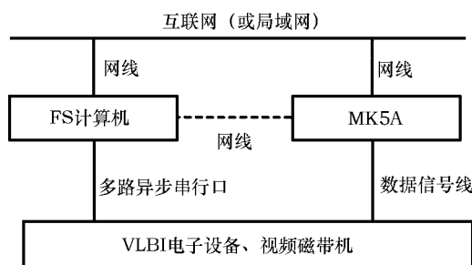
图 1 佘山站 VLBI 终端系统的连接示意图
