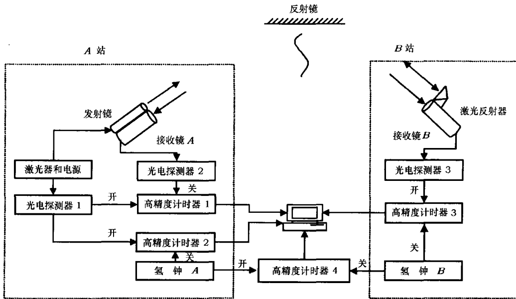
图 6 地面激光时间比对系统框图
